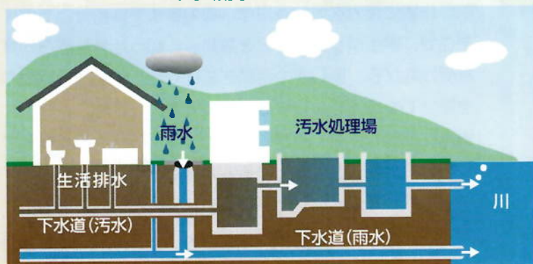
下水(雨水・汚水)の流れ
